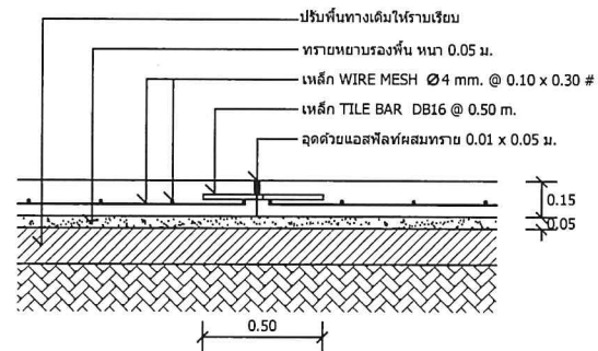
แบบขยาย ค ขยายรอยต่อตามยาว (LONGITUDINAL JOINT) (นายภาณุพงศ์ พรหมจันทร์ วิศวกรโยธา)
