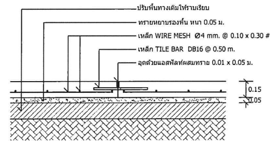
แบบขยาย ข ขยายรอยต่อเพื่อการหดตัว (CONSTRUCTION JOINT) ทุกระยะ 5 เมตร
