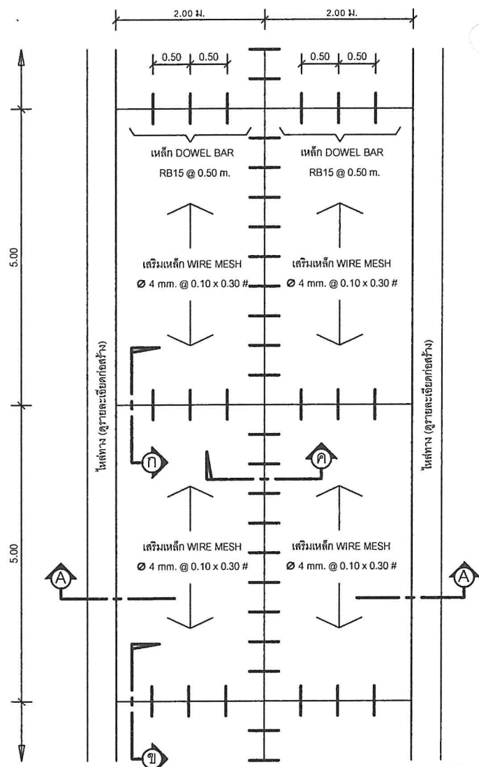
แปลนพื้นถนน
